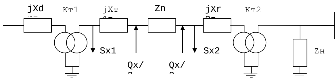
Рисунок 3.5. Схема замещения сети с трансформациями.
